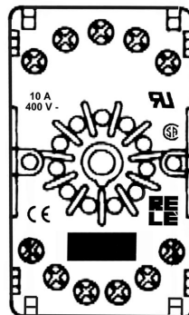
ZVE11 (11-pin)
